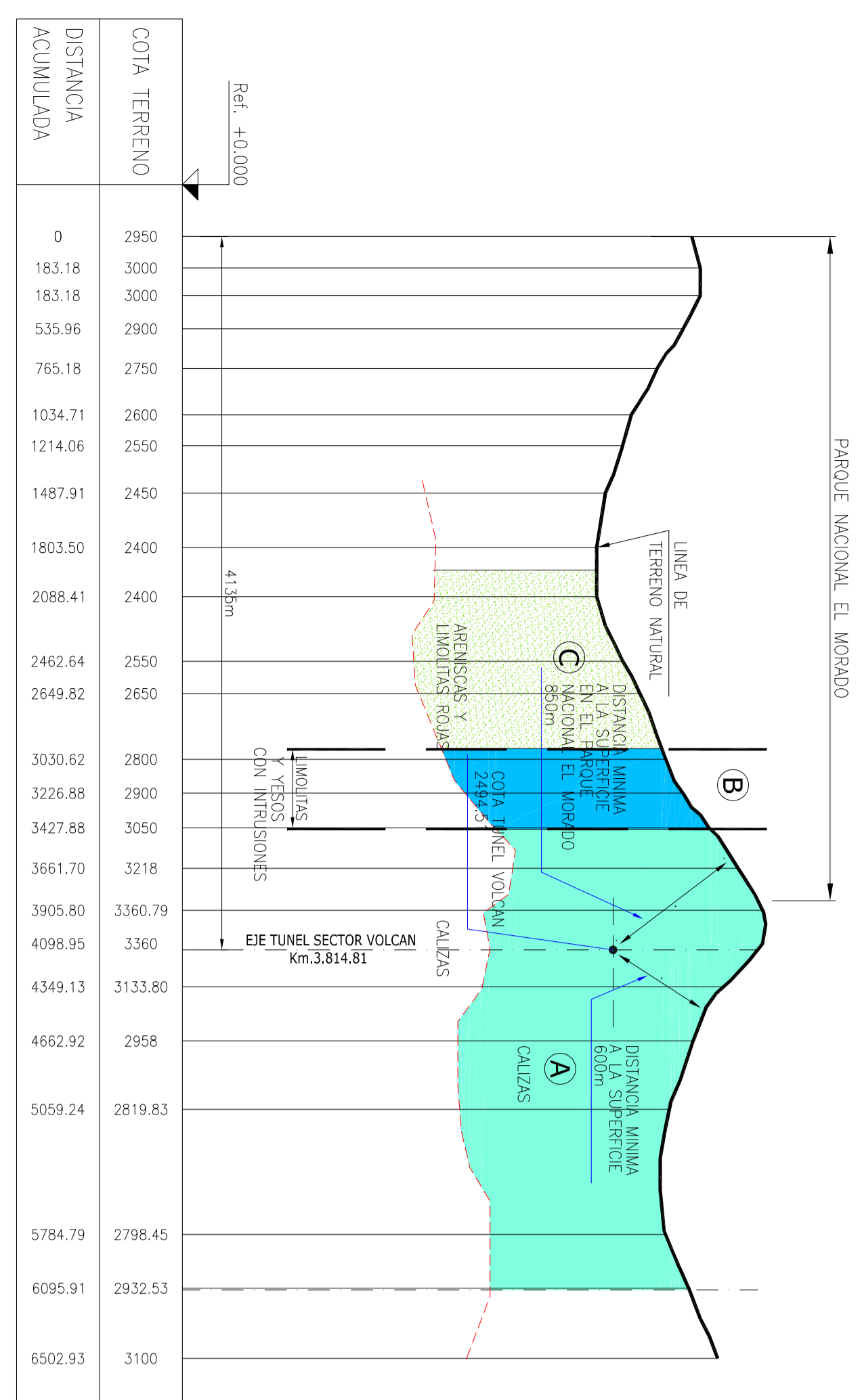
PERFIL 3 Escala Horizontal 1:25000 Escala Vertical 1:25000
