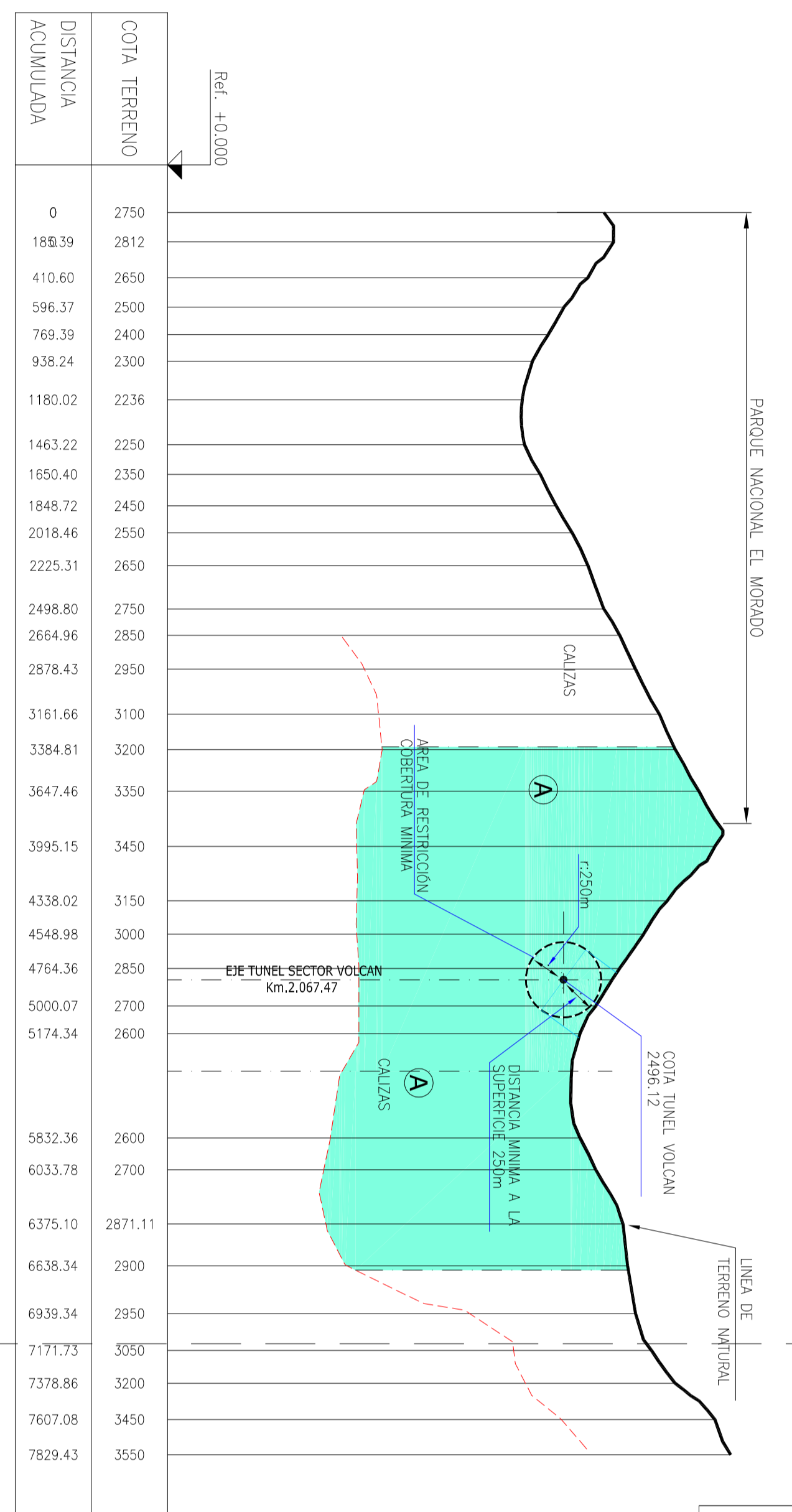
PERFIL 4 Escala Horizontal 1:25000 Escala Vertical 1:25000
