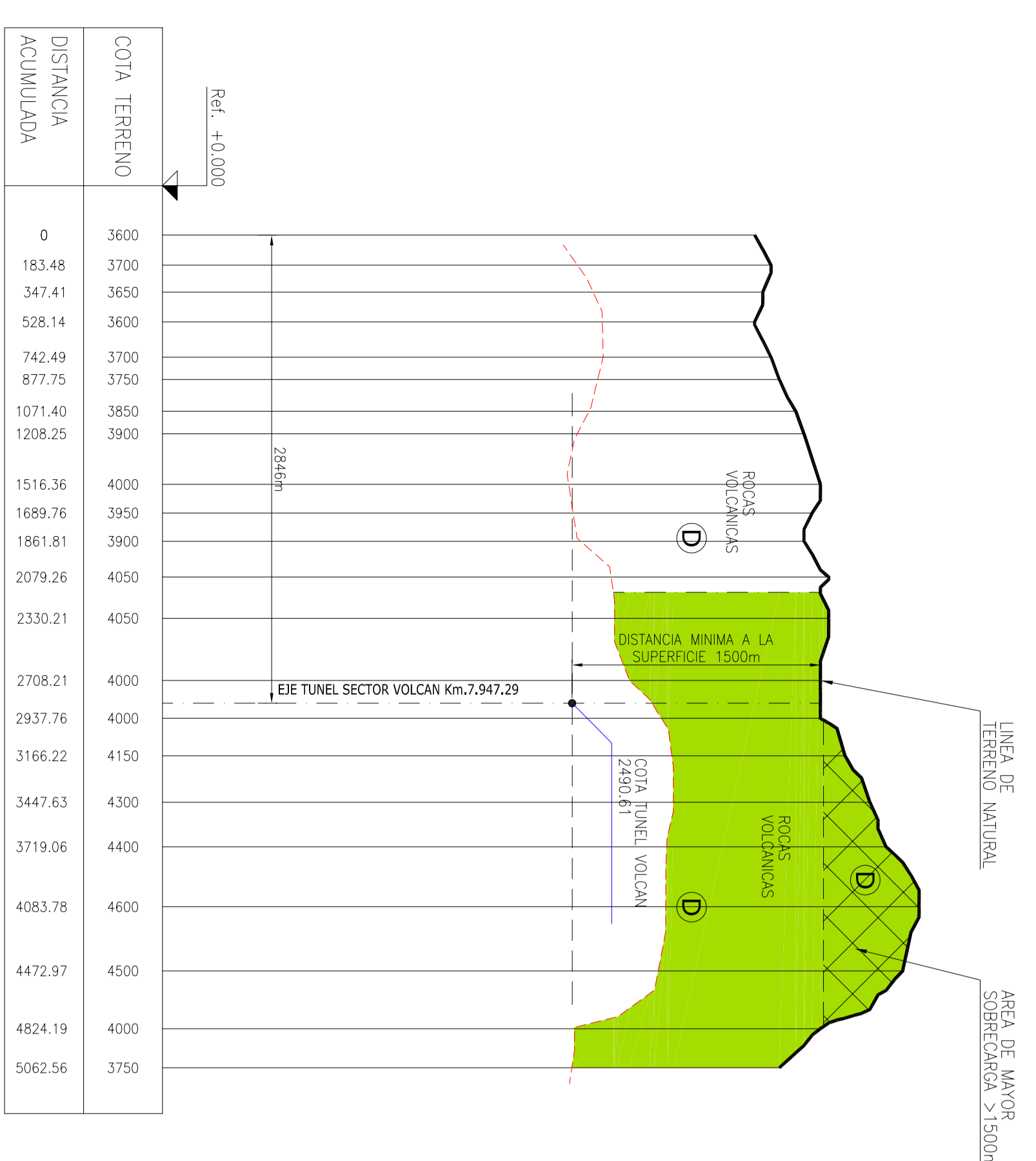
PERFIL 1 Escala Horizontal 1:25000 Escala Vertical 1:25000
