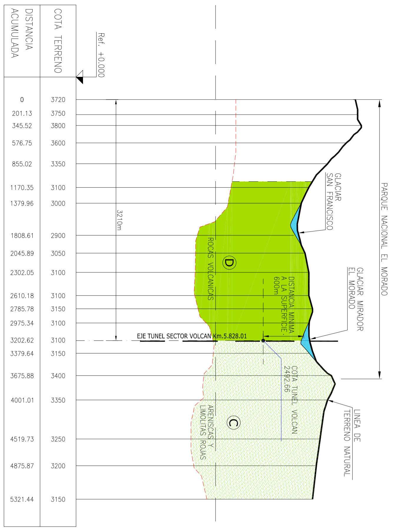
PERFIL 2 Escala Horizontal 1:25000 Escala Vertical 1:25000
